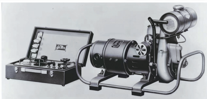
柳州机械厂成功试制出的4马力1101型汽油机
