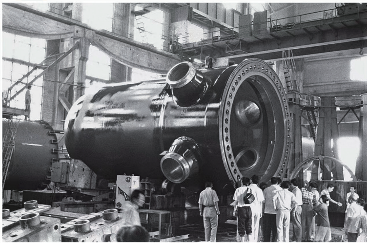
中国第一台 300 兆瓦核电站反应堆压力容器
