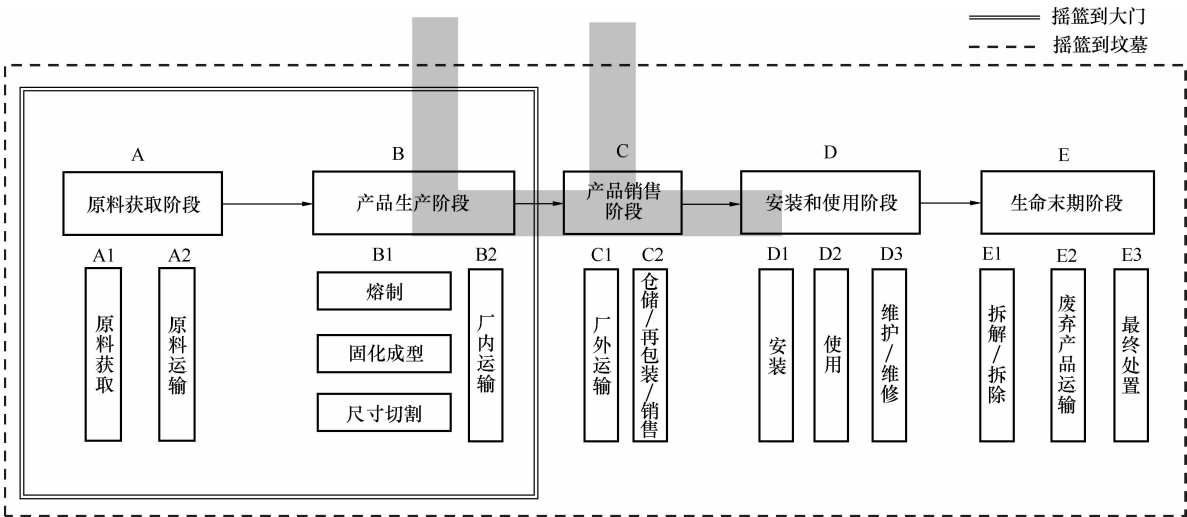
图1 岩（矿）棉及其制品碳足迹评价的系统边界图
