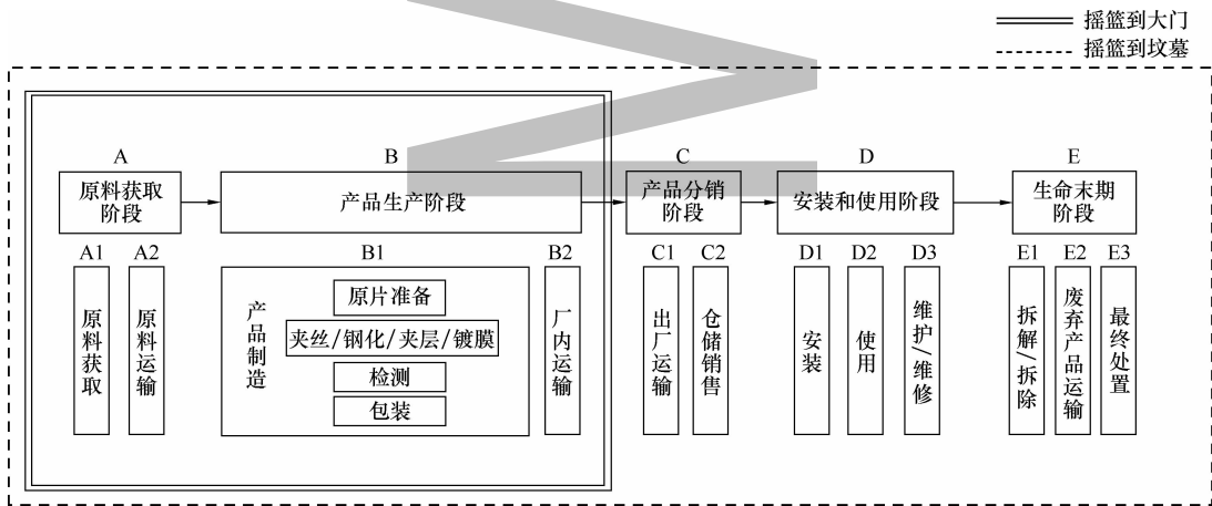
图2 夹丝玻璃、钢化玻璃、夹层玻璃、离线镀膜玻璃碳足迹评价的系统边界图
