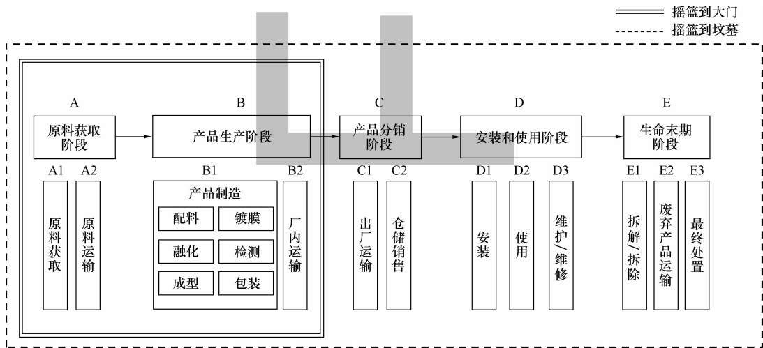
图1 浮法玻璃、溢流玻璃、压延玻璃、在线镀膜玻璃碳足迹评价的系统边界图
