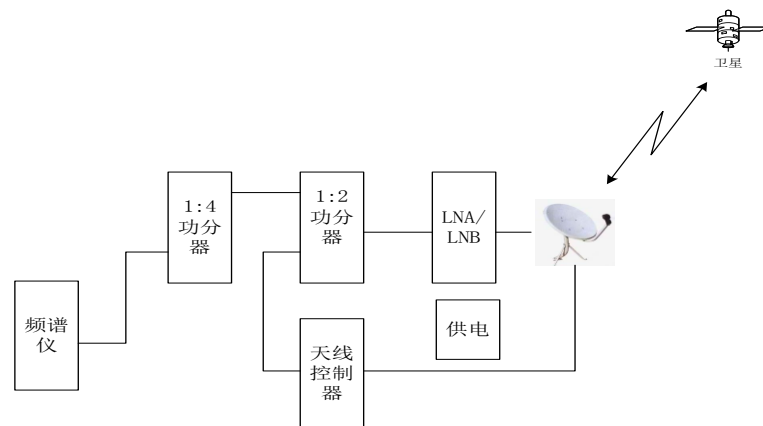
图 4.2.3 寻星控制测试框图
