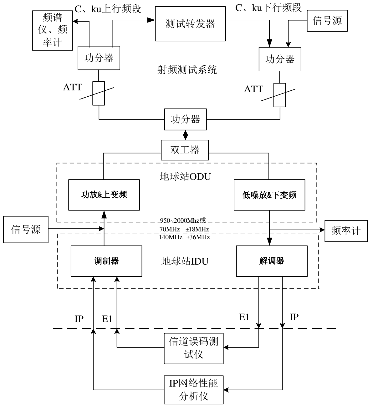
卫星地球站室射频环路测试系统图
