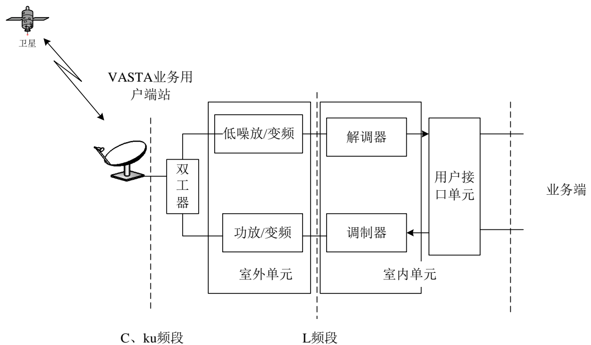
图 3.0.1 VSAT 卫星地球站设备组成框图
