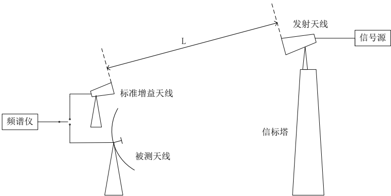
图 4.3.1 天线方向图测试原理示意图
